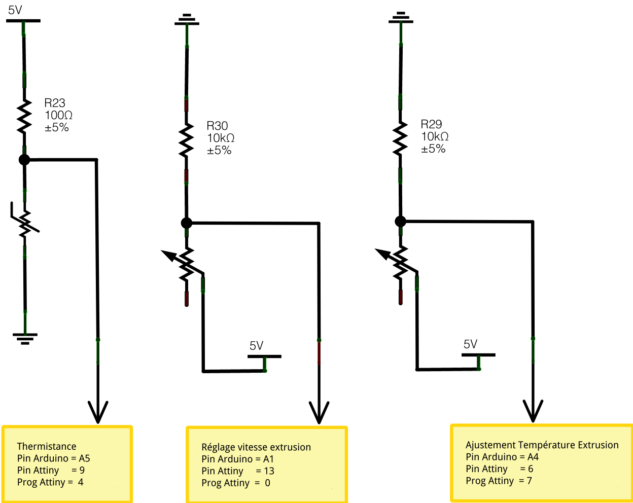
REGLAGE VITESSE FIL ET TEMPERATURE EXTRUSION
