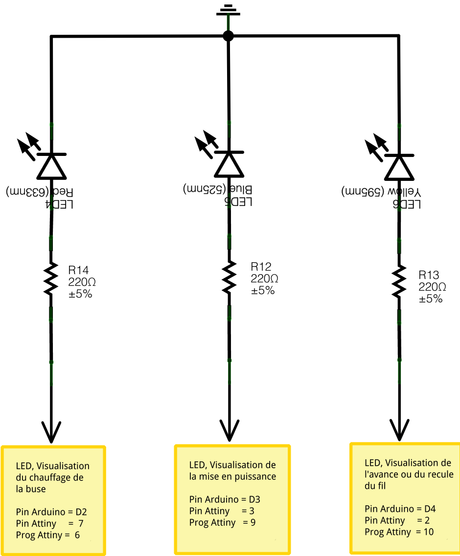
VISUALISATION DU FONCTIONNEMENT DU STYLO 3D
