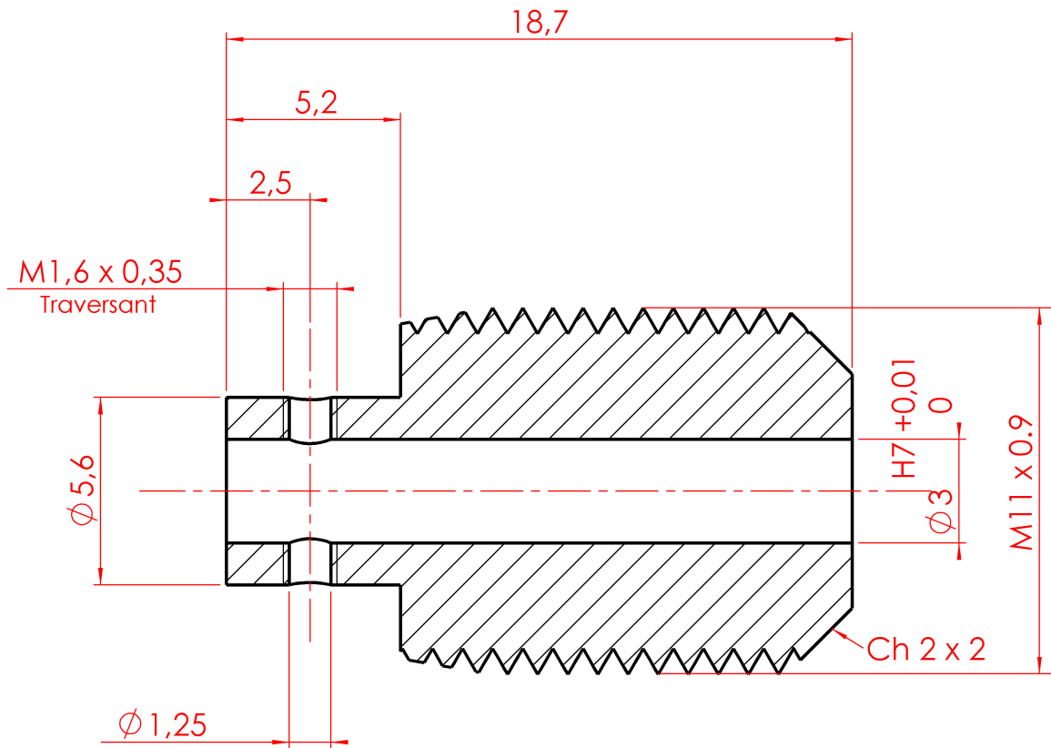
COUPE A-A ECHELLE 5 : 1
