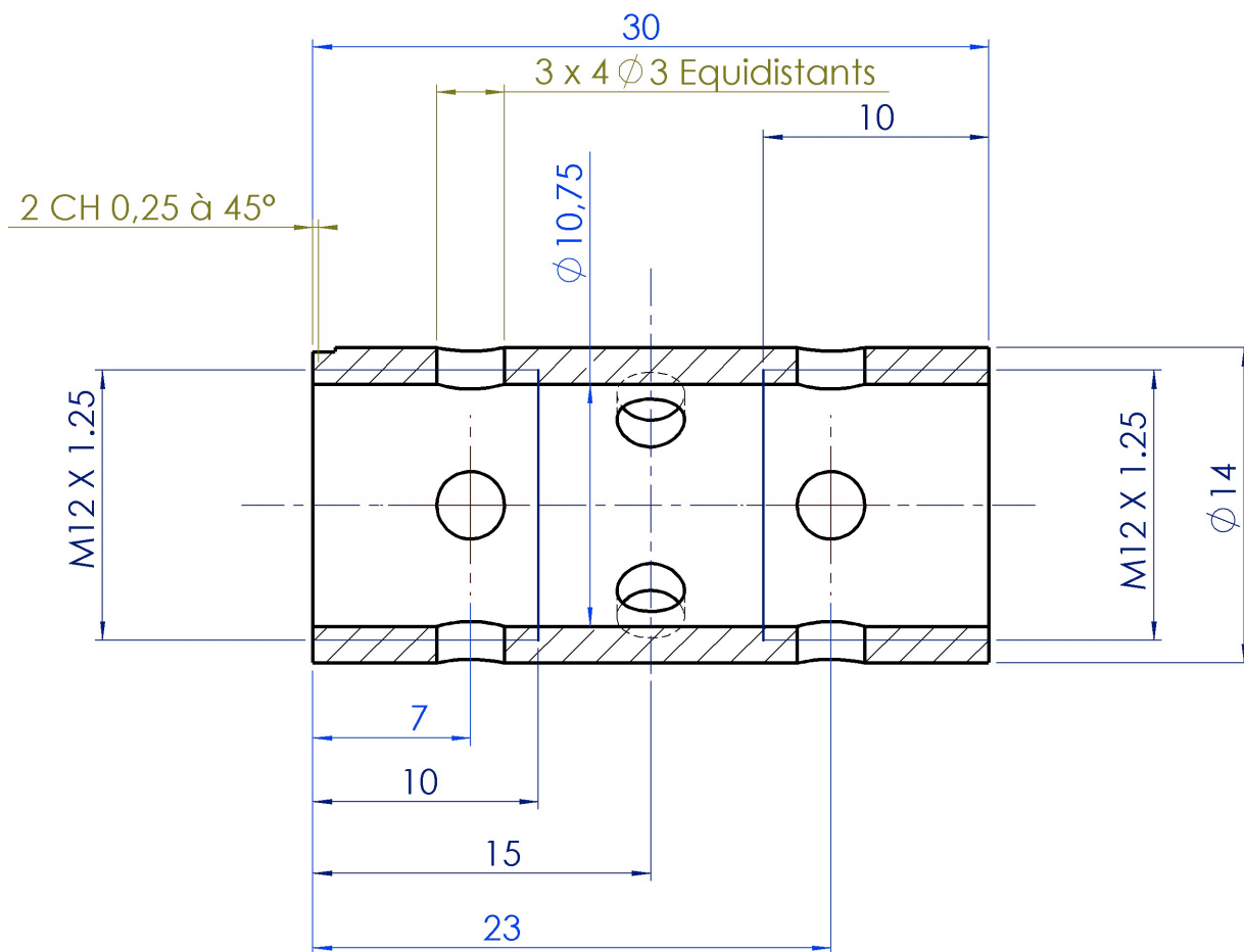
COUPE A-A ECHELLE 3:1
