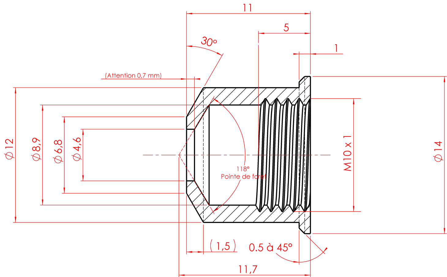
COUPE A-A ECHELLE 5 : 1
