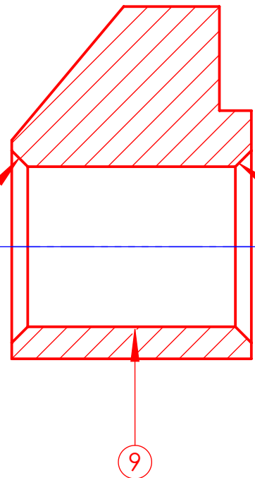
COUPE A-A Echelle: 3/1
