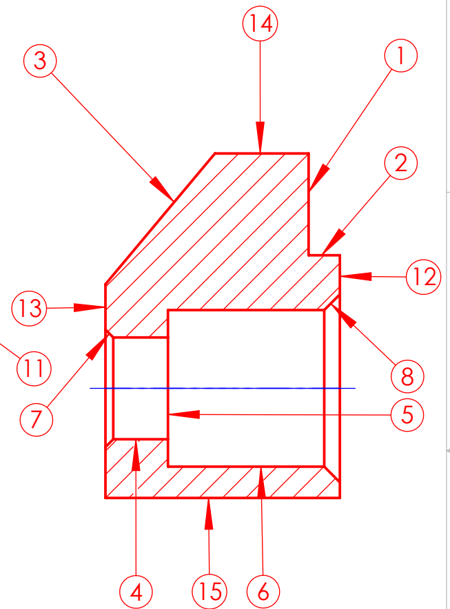
COUPE B-B Echelle: 3/1
